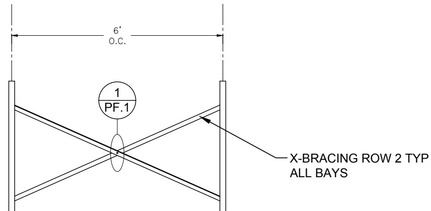
FRAME SECTION SCALE: NTS
